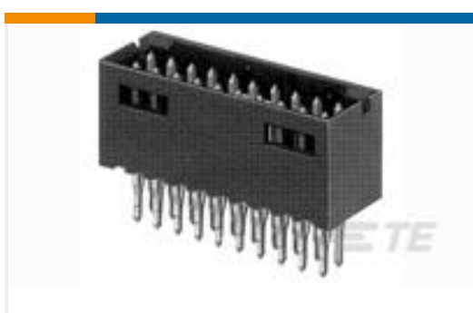
TE 零件编号1-102699-2 26 MODII HDR DRST SHRD A/PIN
